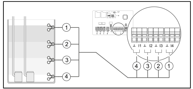
Abb. 1: Schwimmerschalter Duo
