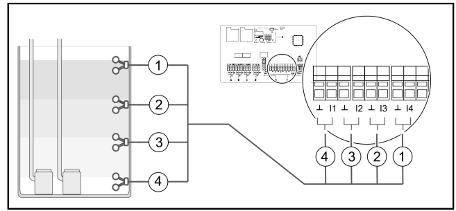
Afb. 1: Vlotterschakelaar Duo
